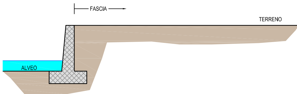
ARGINE IN CEMENTO ARMATO DISTANZA MISURATA A PARTIRE DAL CIGLIO ESTERNO (SOMMITA') DEL MANUFATTO
