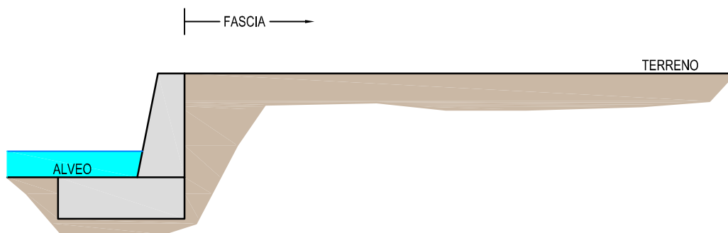
ARGINE IN CALCESTRUZZO DISTANZA MISURATA A PARTIRE DAL CIGLIO ESTERNO (SOMMITA') DEL MANUFATTO
