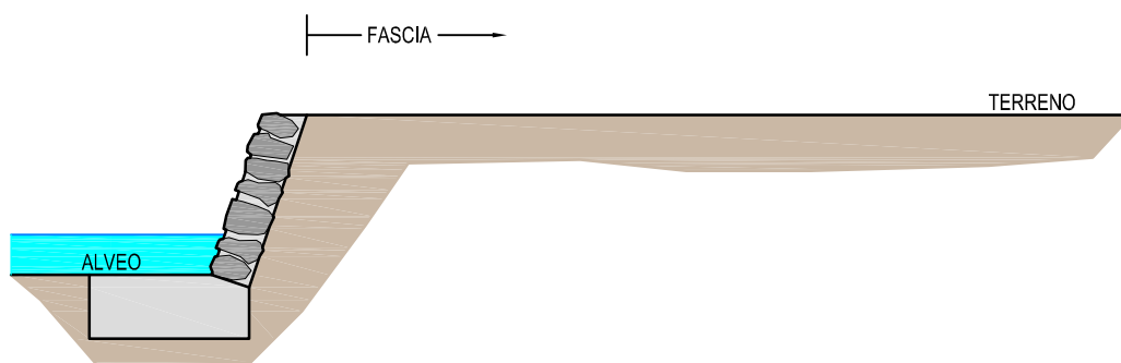
ARGINE IN PIETrame E MALTA DISTANZA MISURATA A PARTIRE DAL CIGLIO ESTERNO (SOMMITA') DEL MANUFATTO
